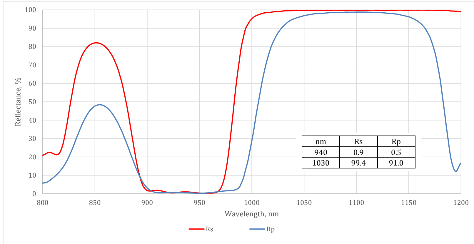
Reflectance, s, p polarization AOI=45 deg
